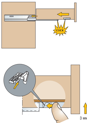
Схема сборки и регулировки
